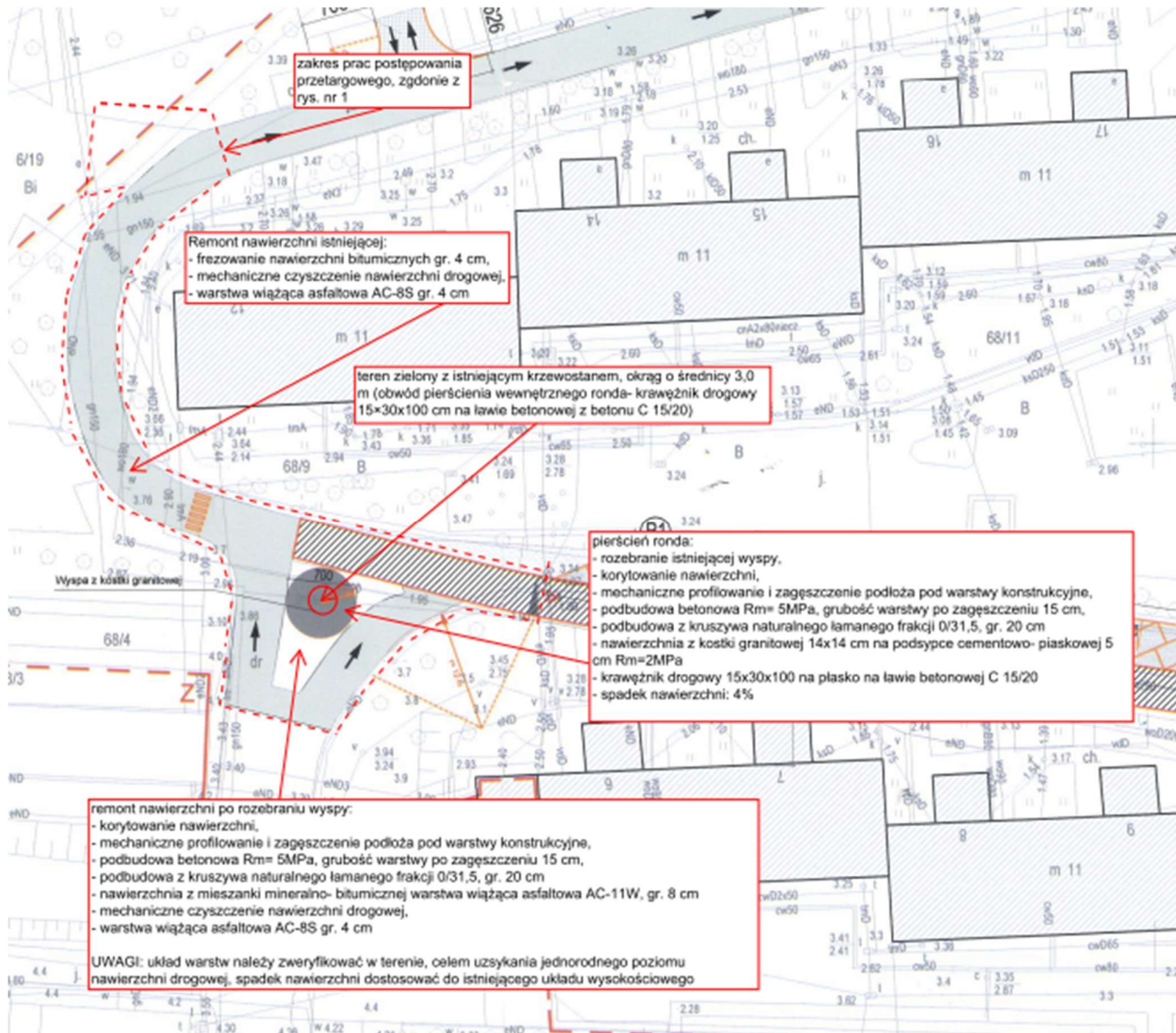
Rys. nr 2 – wycinek dokumentacji projektowej z graficznym zestawieniem zakresu robót
