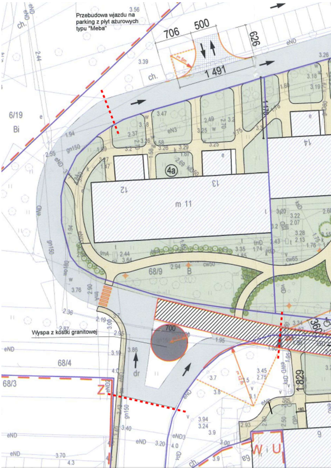
Rys. nr 3 – wycinek dokumentacji projektowej „Projekt zagospodarowania terenu”
